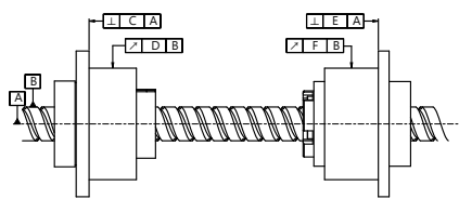
RFBY回転式ナット
